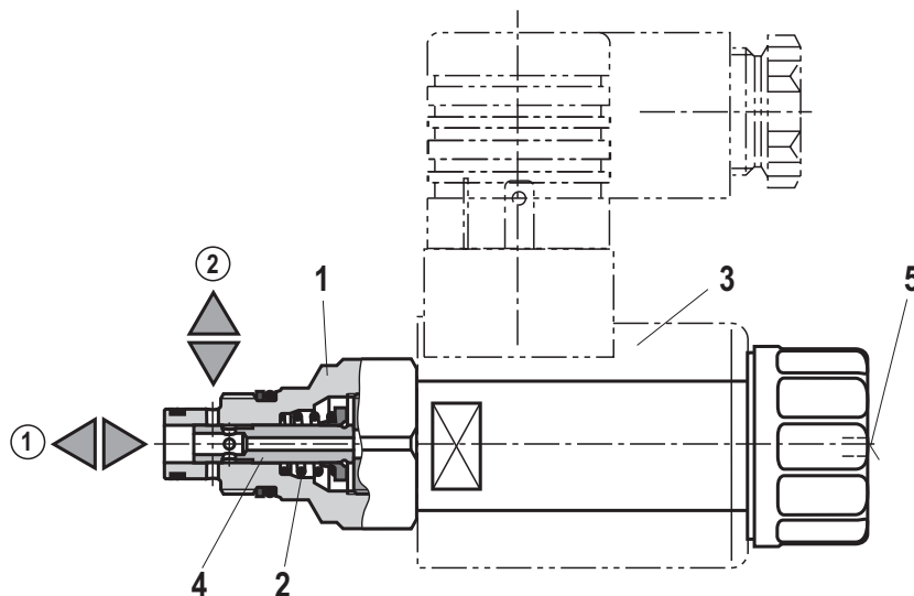
Ausführung „K4“ (mit Leitungsdose)
